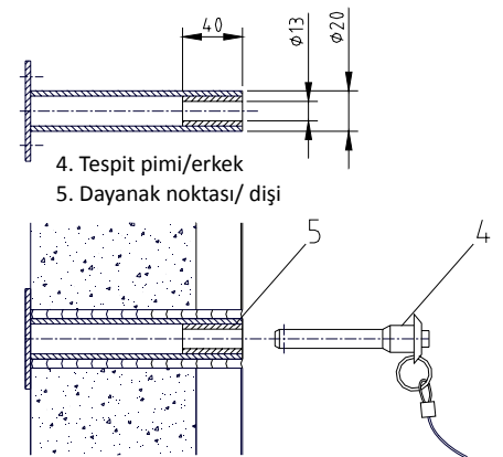
Önerilen Tutunma Sistemi
