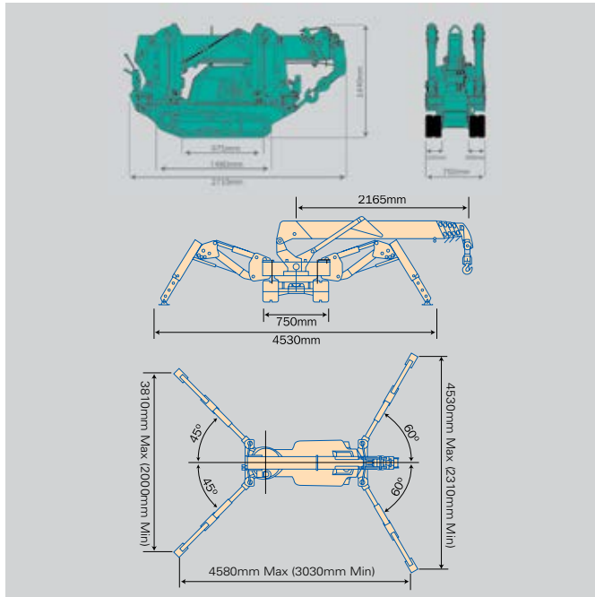
Diyagramda destek bacakları maksimum konumlarında gösterilmiştir
