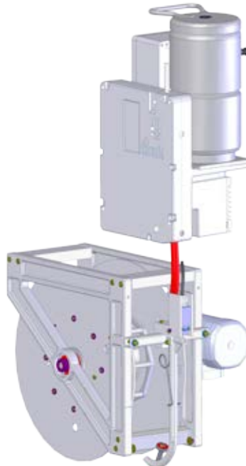
Ayrı hareket ettirilen çelik halat makarası
