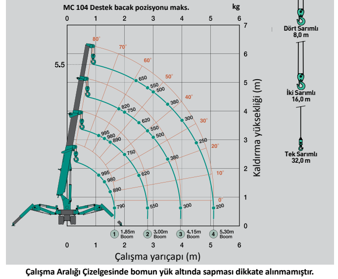
Çalışma Aralığı Çizelgesinde bomun yük altında saptması dikkate alınmamıştır.
