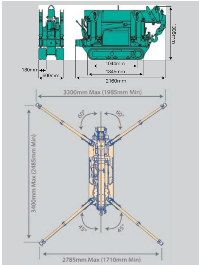
Diyagramda destek bacakları maksimum konumlarında gösterilmiştir
