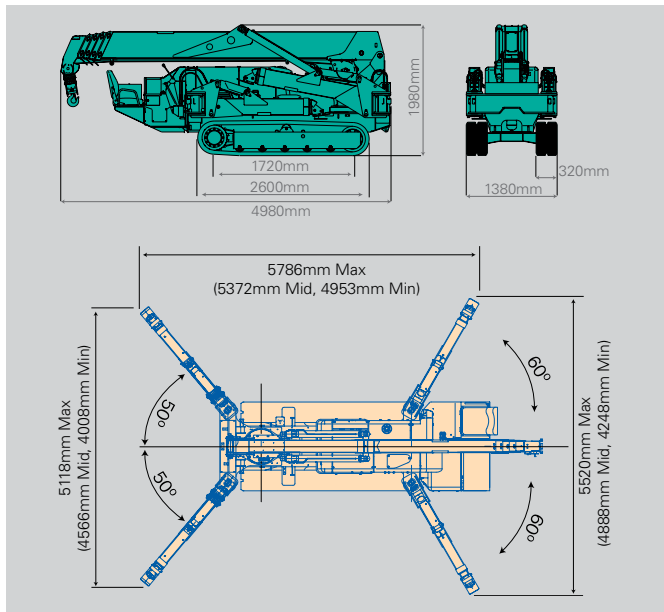
Diyagramda destek bacakları maksimum konumlarında gösterilmiştir
